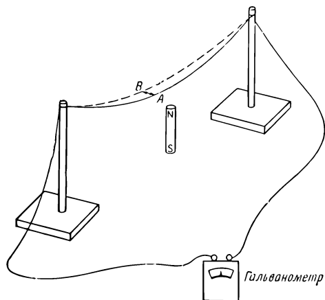
Фиг. 16.2. Движение провода в магнитном поле создает ток (это регистрирует гальванометр).
