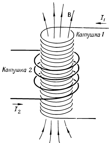
Ф и г. 17.8. Ток в катушке 1 создает магнитное поле, проходящее через катушку 2.
