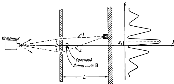
Ф и г. 15.7. Магнитное поле способно влиять на движение электронов, даже когда оно существует только в области, где вероятность обнаружить электрон пренебрежимо мала.
