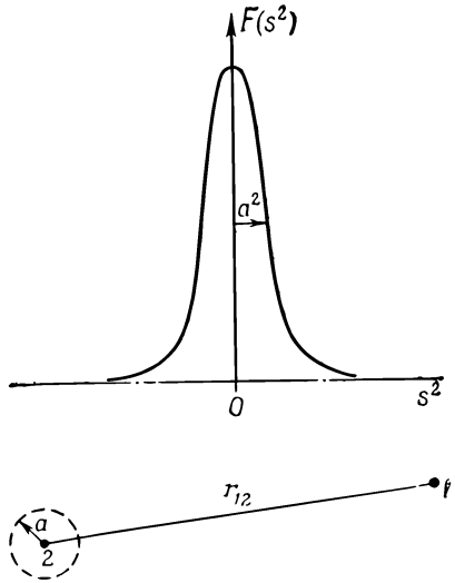
Фиг. 28.4. Функция F(s^2) , используемая в нелокальной теории Боппа.
