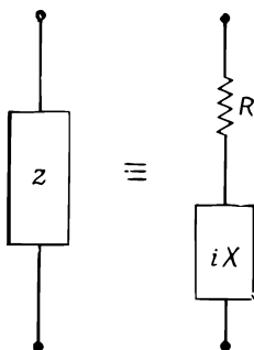
Фиг. 22.17 Любой импеданс эквивалентен последовательному соединению чистого сопротивления и чистого реактанса.
