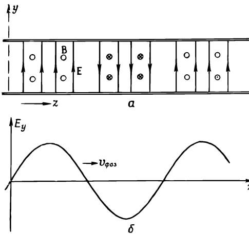
Фиг. 24.5. Зависимость поля в волноводе от z .
