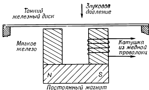
Ф и г. 16.4. Приемное или передающее устройство телефона.
