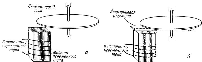
Ф и г. 16.15. Простой пример индукционного мотора затененным полюсом.
