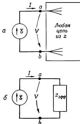
Фиг. 22.15. Любая сеть пассивных элементов с двумя выводами эквивалентна эффективному импедансу.
