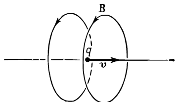
Фиг. 26.5. Магнитное поле вблизи движущегося заряда равно \mathbf{v} \times \mathbf{E} (ср. с фиг. 26.4).
