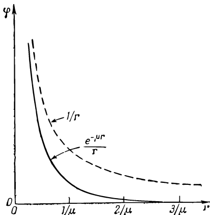
Фиг. 28.6. Сравнение потенциала Юкавы e^{-\mu r}/r с кулоновым потенциалом 1/r .
