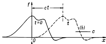
Фиг. 20.4. Функция f(x - ct) представляет неизменный «коптур», движущийся в направлении возрастания x со скоростью c .
