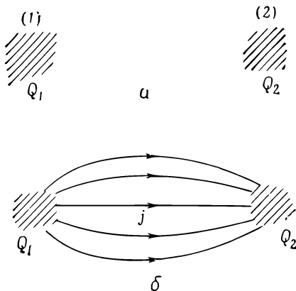
Фиг. 27.1. Два способа описания сохранения заряда. а: Q_1 + Q_2 постоянно.
