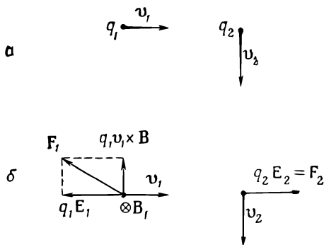
Фиг. 26.6. Силы между двумя движущимися зарядами не всегда равны и противоположны. «Действие», оказывается, не равно «противодействию».
