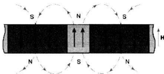
Рис. 6.8.5. Перпендикулярная запись информации на образцах с осью легкого намагничивания, направленной перпендикулярно их поверхности. В средней части рабочего слоя носителя находится перемагниченный участок
