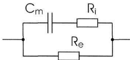
Рис. 8.4.5. Эквивалентная электрическая схема живой клетки и ее окружения.
