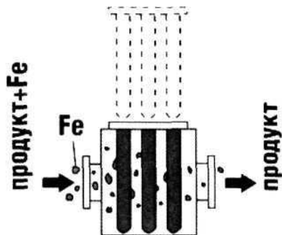
Схема 1. Принцип работы СМТП
