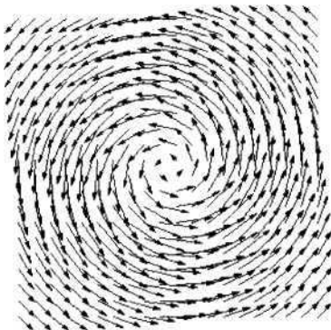
Рис.4.11.11. Картина векторного поля плотности вихревого тока от катушки Рис.4.11.9 в слое проводящей среды на глубине 3 см
