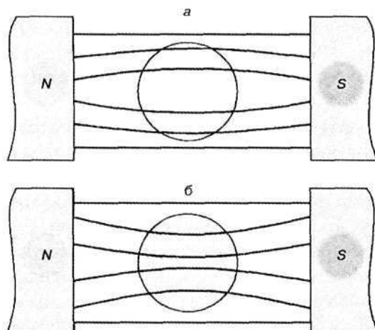
Рис. 4.7.1. Поведение различных веществ в магнитном поле: а -- диамагнетики, б -- парамагнетики
