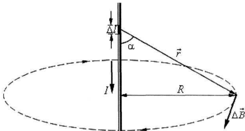
Рис. 2.2.1. Иллюстрация закона Био-Савара
