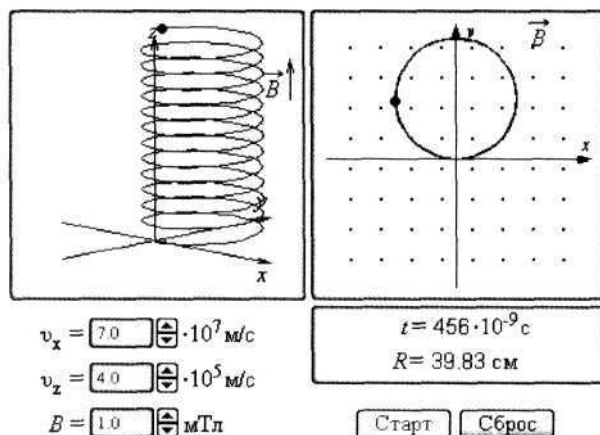
Модель. Движение заряда в магнитном поле
