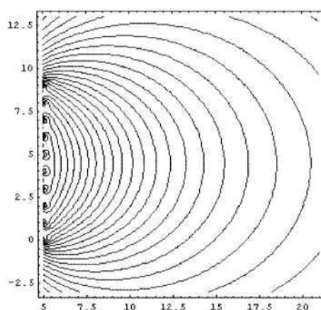
Рис.4.11.9. Картина силовых линий магнитной индукции для вертикальной катушки из 10 витков. Центр нижнего витка расположен в начале координат. Расстояния даны в см
