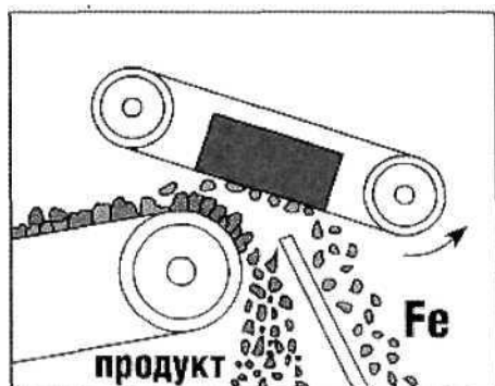
Схема 2. Способ установки № 2
