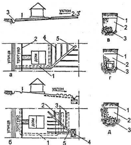
Рис. 4. Осушение участка:
