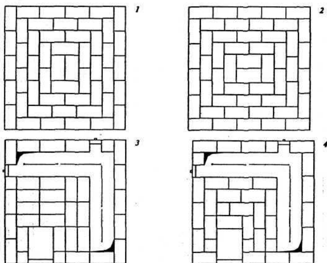
Рис. 12. Порядовка банной печи-каменки № 3
